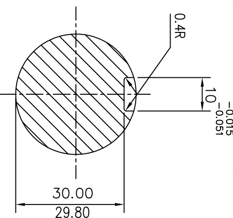
KEYWAY DETAIL (INPUT) --R10:1
